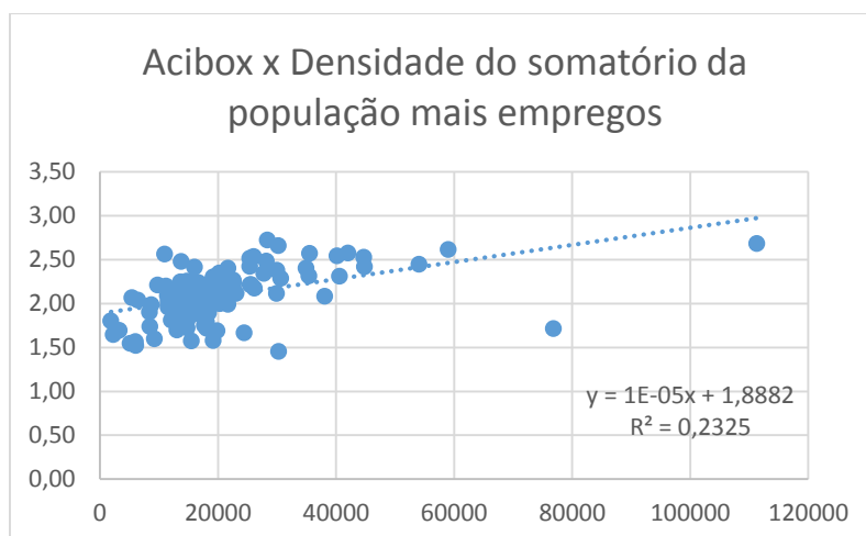
Figura 43 Gráfico da densidade de acidentes com transformação de Box e Cox versus somatório da população mais empregos
