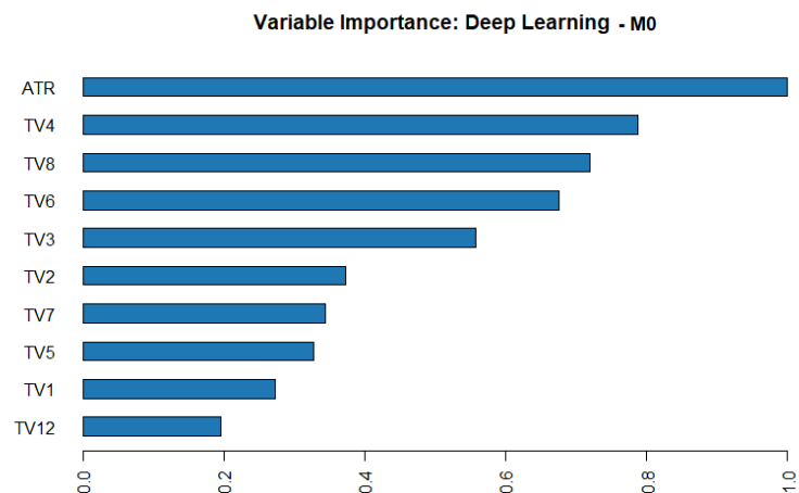
Figura 5.4. Significância das variáveis em M0 (30-100). Elaboração própria.
