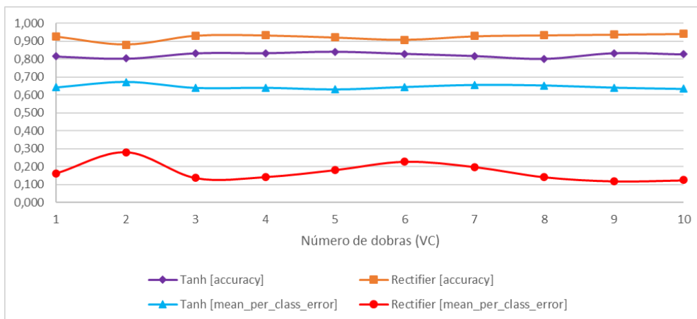
Figura 4.7. Avaliação da função de ativação. Elaboração própria.
