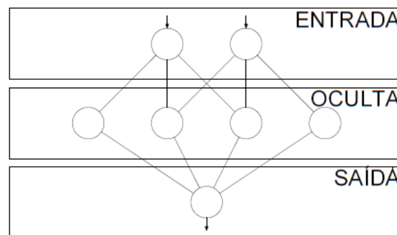
Figura 2.2. Estrutura da rede neural.
