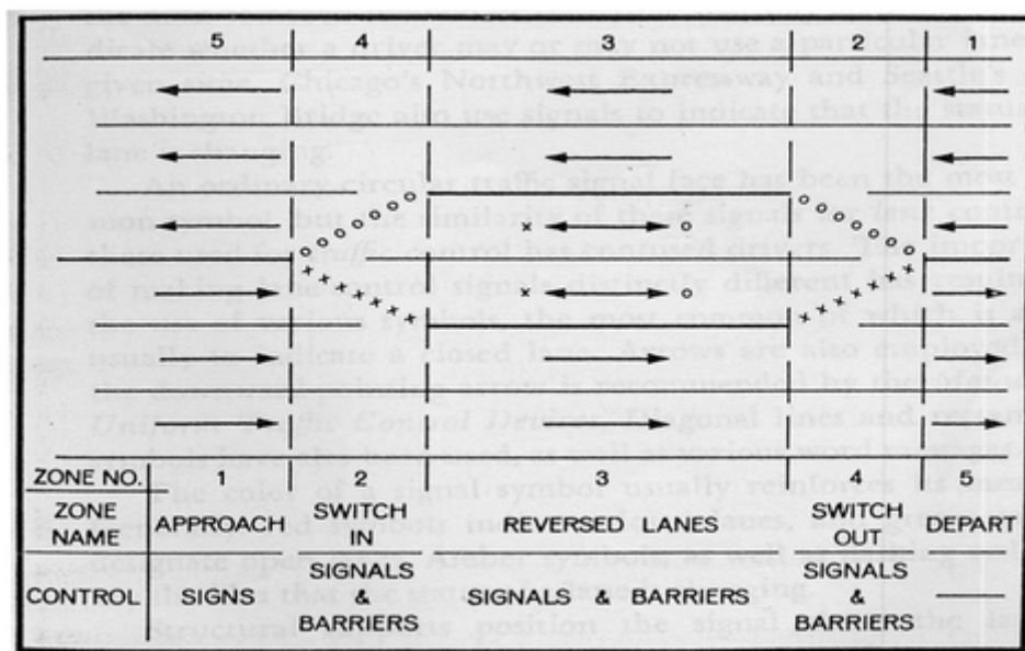
Figura 1: Configuração geral das operações de pistas reversíveis (Lathrop 1972).
