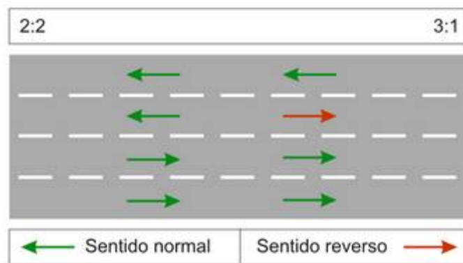
Figura 4: Configuração das alterações de operações reversíveis de 2:2 para 3:1.
