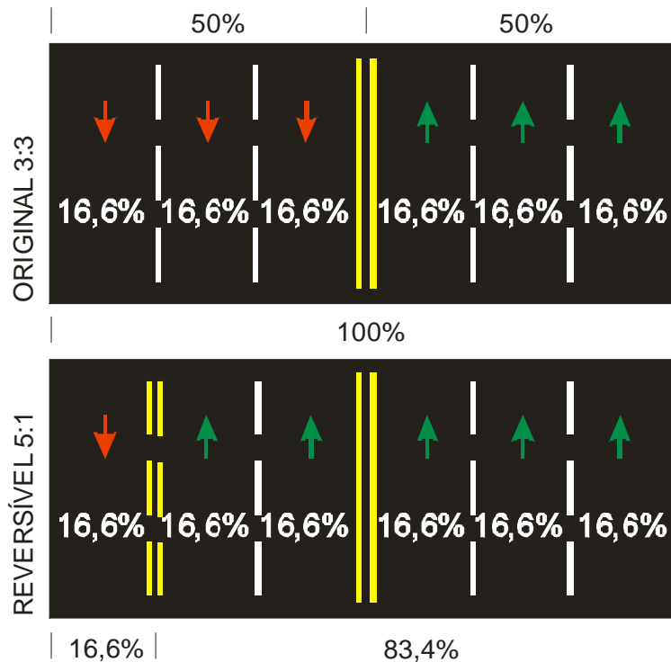
Figura 18: Configuração 3:3 – 5:1 com percentuais associados à capacidade.
