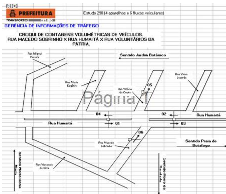
Figura 24: Pontos de contagens volumétricas da CET Rio.
