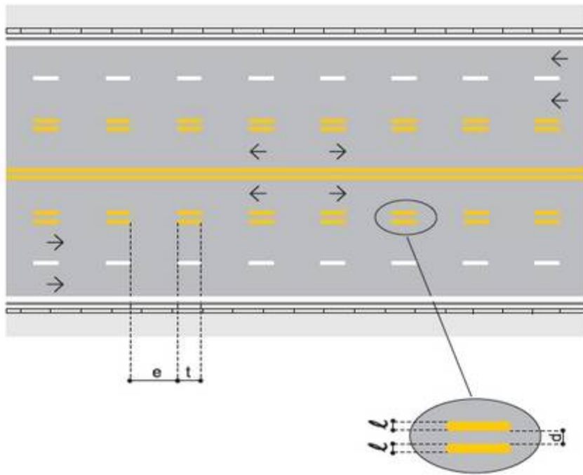
Figura 12: Relação entre largura, espaço, cadência e traço para faixas reversíveis.
