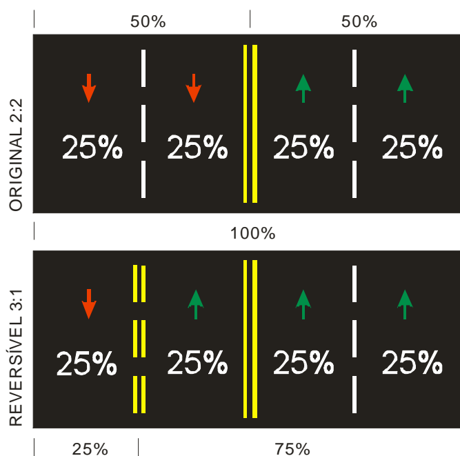
Figura 16: Configuração 2:2 – 3:1 com percentuais associados ao volume de tráfego.
