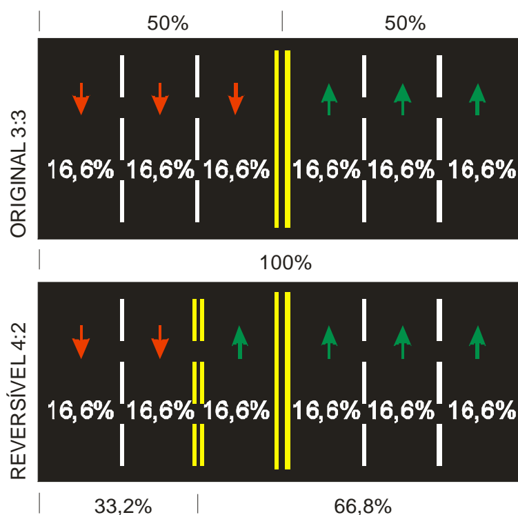
Figura 17: Configuração 3:3 – 4:2 com percentuais associados à capacidade.
